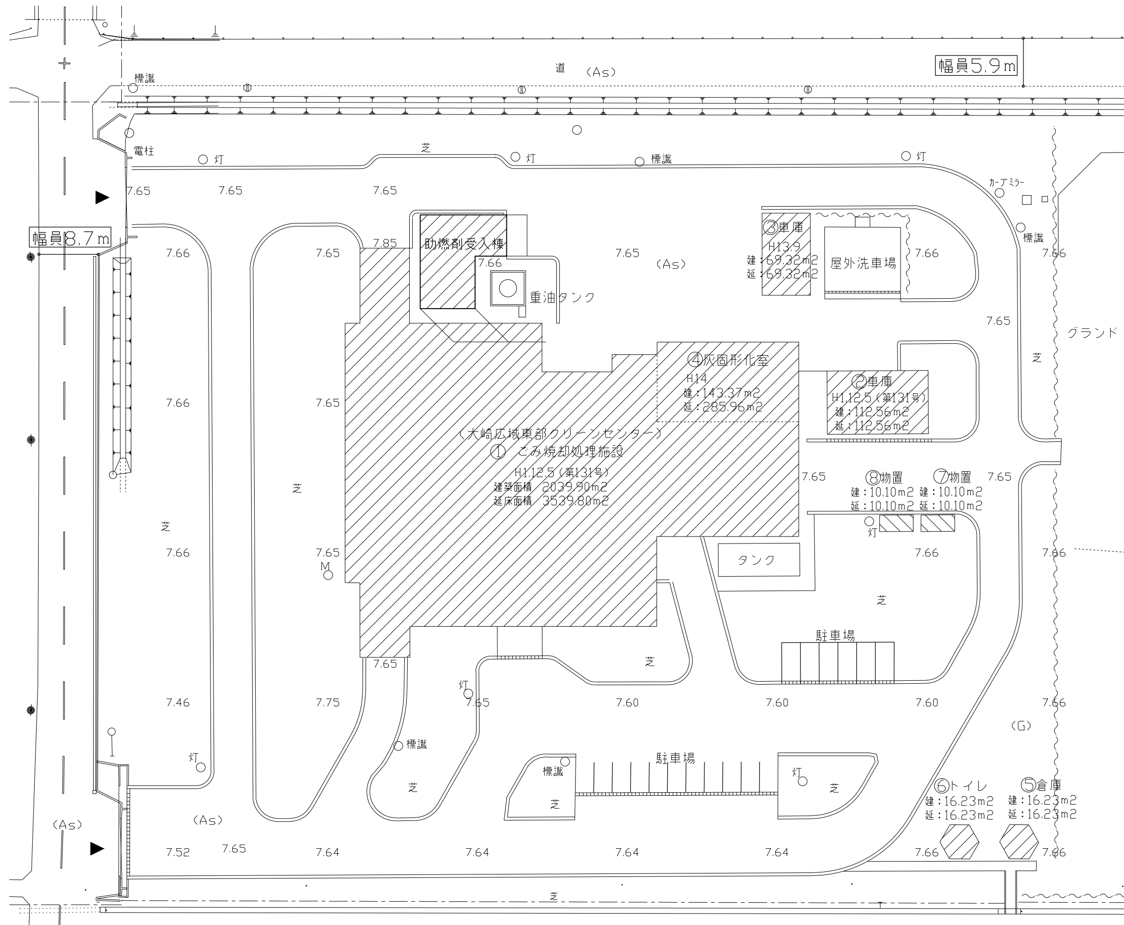
既設 S=1:500
